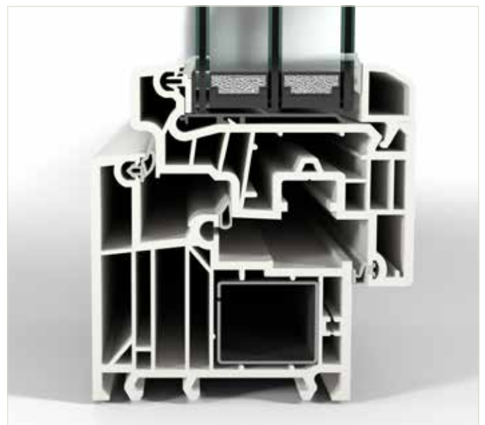
doorsnede van kunststof raamwerk van Finstral: FIN-Window Slim-line 77 kunststof-kunststof
