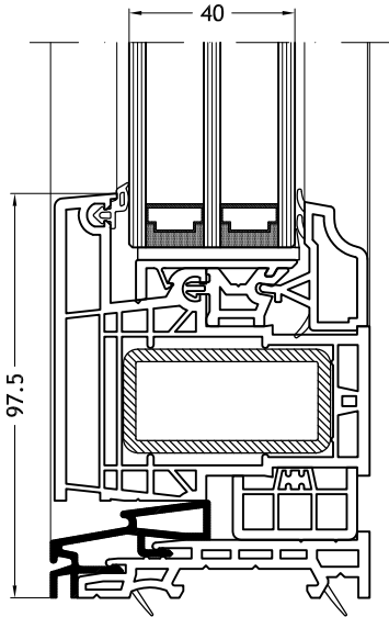
Vlakke onderdorpel met vast raam met glaslat stijl
